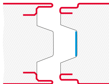
połączenie w systemie nakładkowo-zakładkowym
